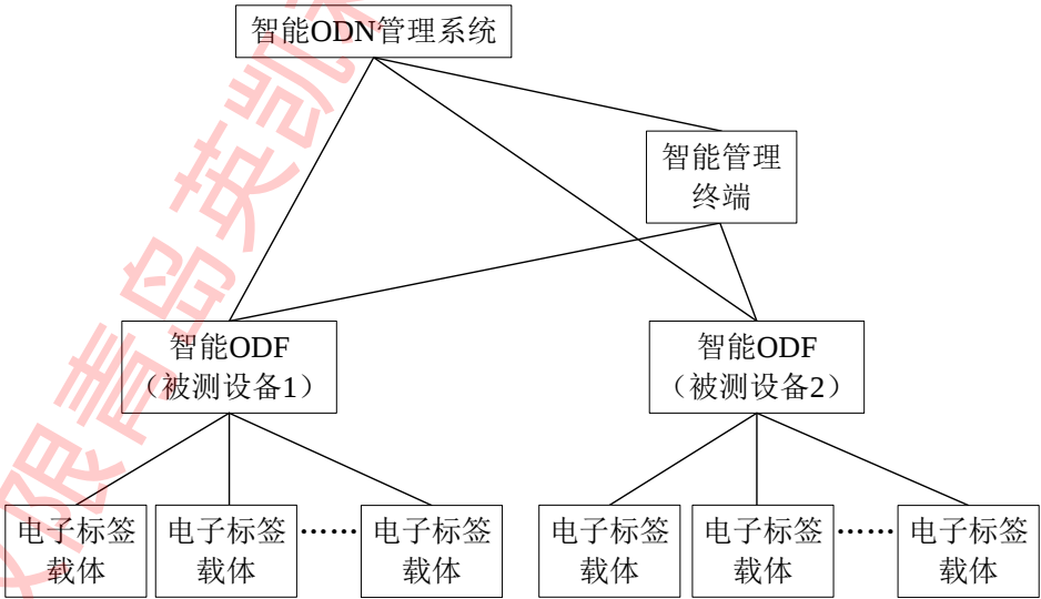
图 3 智能 ODF 的测试示意图
