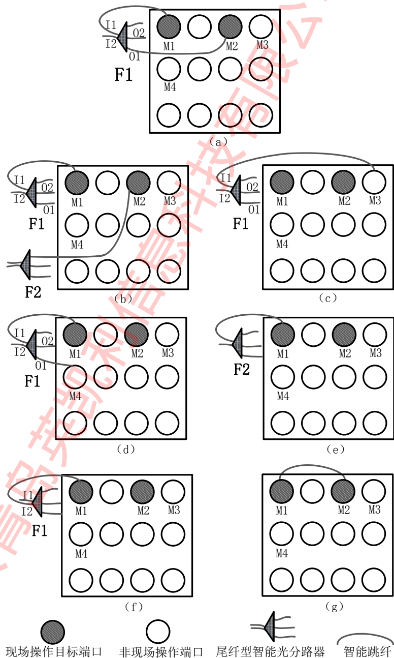
图 5 尾纤型智能光分路器的端口光纤跳接错误指示测试示意图
