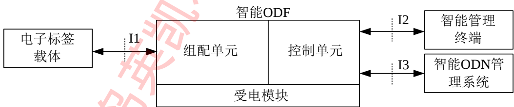
图 1 智能 ODF 逻辑组成示意图
