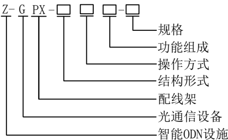
图 2 智能 ODF 型号
